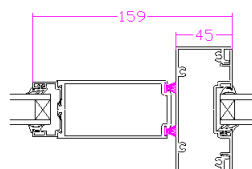
DETAIL E - E
